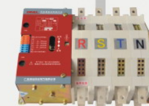
双电源自动转换开关 DNQ8-200(4P)
